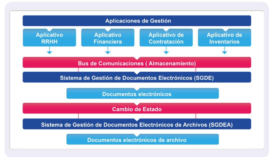
Ilustración 3. Integración del Gestor de Documentos. Fuente: Elaboración propia.
